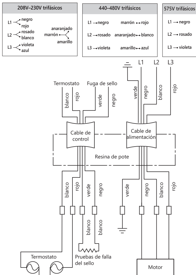
Figura 2. Diagrama de cableado trifásico
